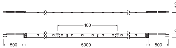
Voorbedrade kabels aan beide zijden
