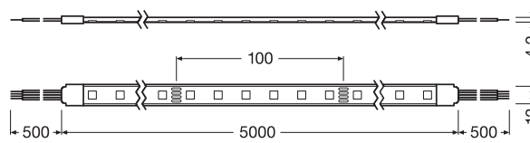
Voorbedrade kabels aan beide zijden
