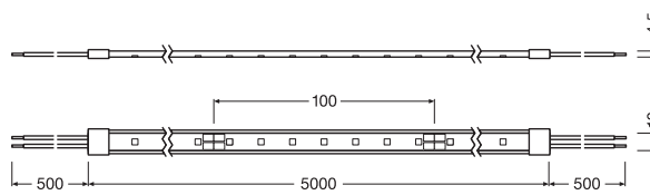
Voorbedrade kabels aan beide zijden
