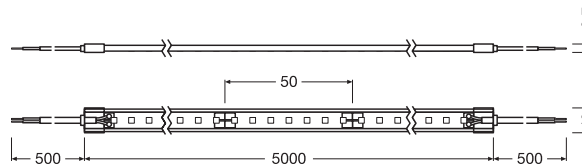
Voorbedrade kabels aan beide zijden
